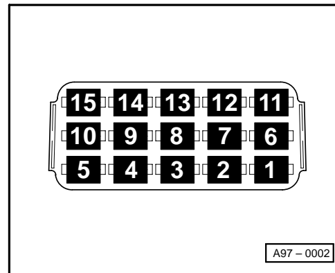
Relaisträger E-Box Beifahrerfußraum
