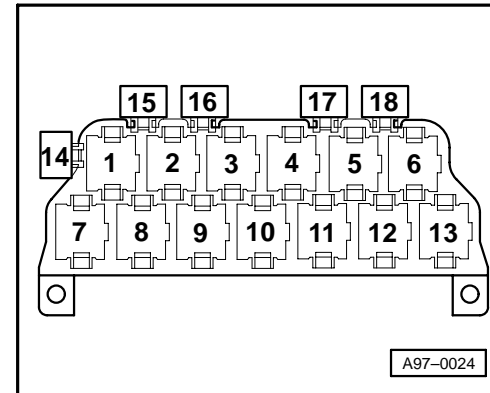
13-fach Relaisträger
