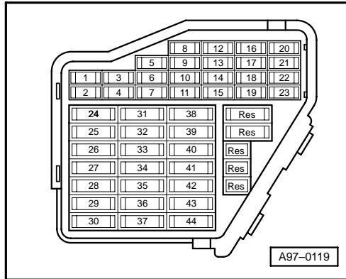
Sicherungshalter
