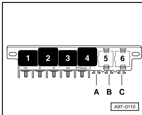
Mikrozentralelektrik
